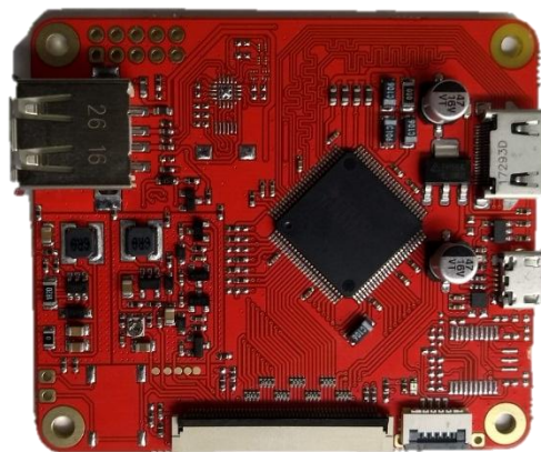
Display TFT com entrada HDMI
